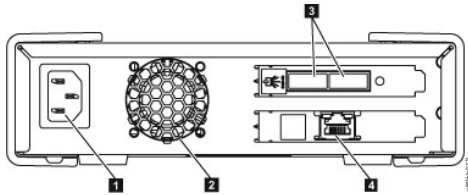
図 5. 外付け SAS テープ・ドライブの背面パネル
