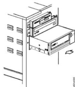
図 7. ドライブを取り付ける
