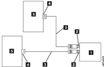
図 12. 2 つの SAS デバイスの接続
