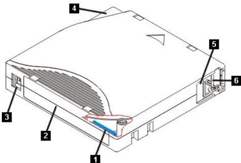
図 14. LTO Ultrium 1500 GB データ・カートリッジ
